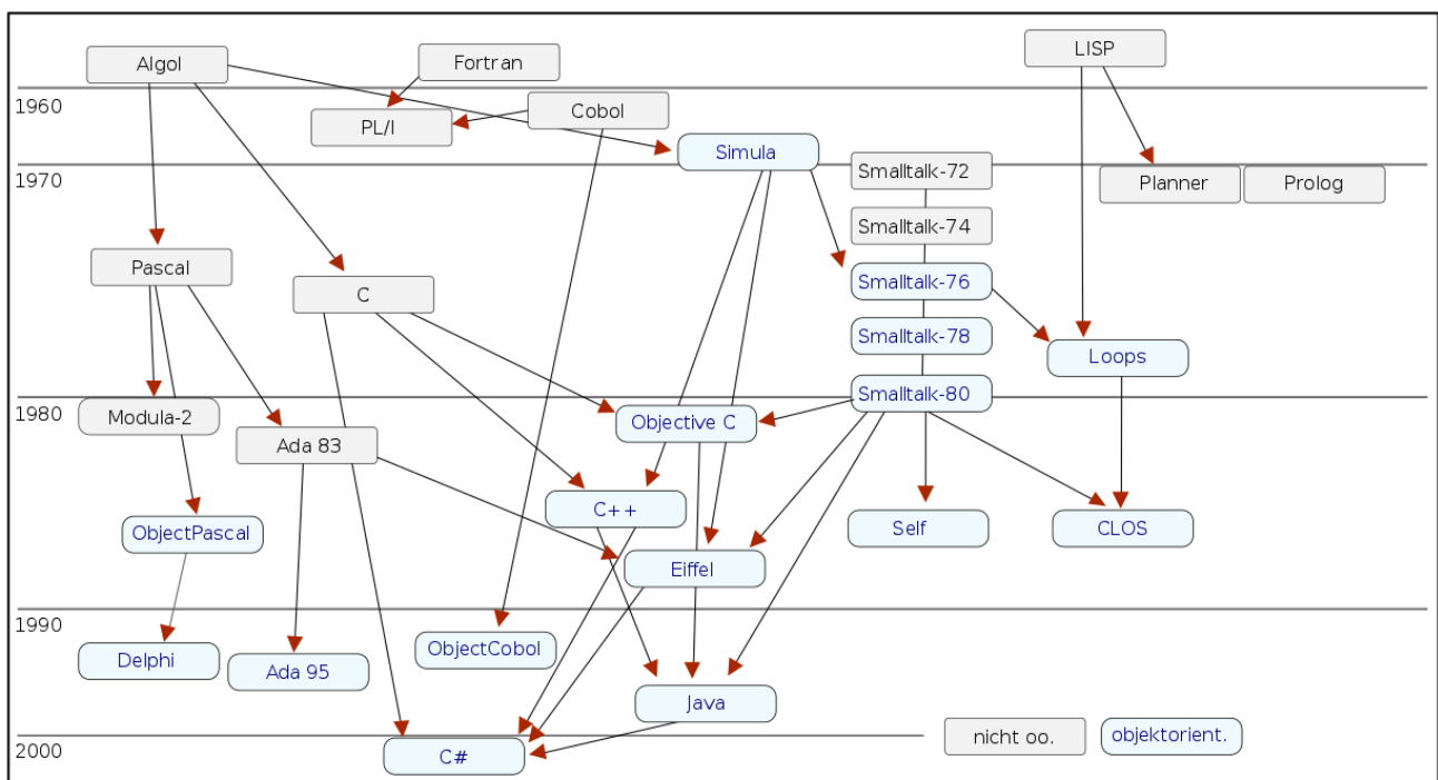
Darstellung der Entwicklung von objektorientierten/nicht-objektorientierten Programmiersprachen [1]
